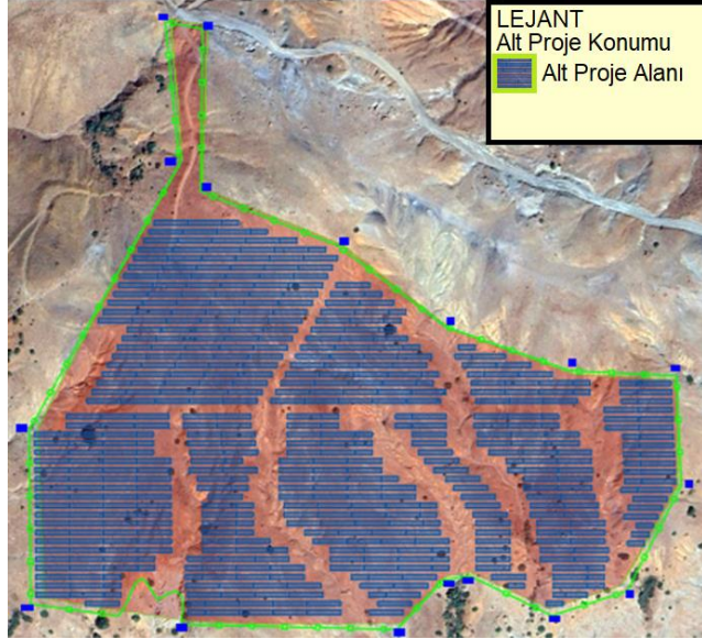
Şekil 1: Ümraniye GES Proje Alanı
