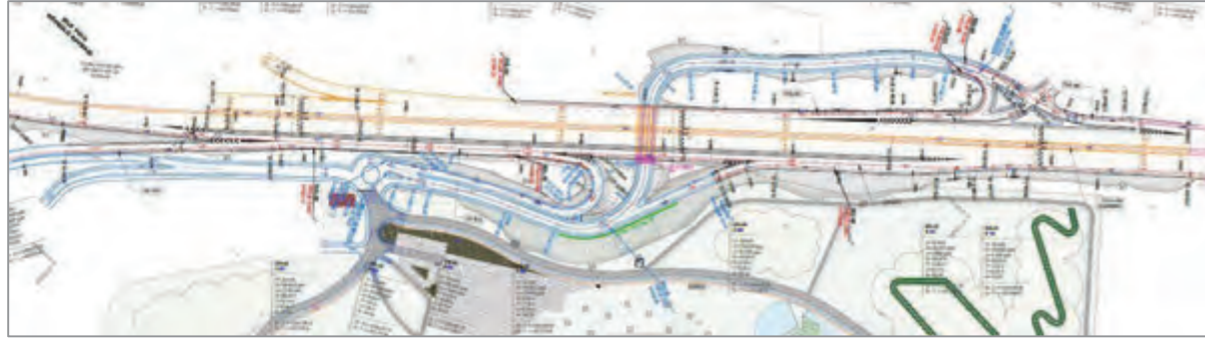
Şile Otoyolu Trabzon Park Millet Bahçesi Trafik Giriş-Çıkış Düzenleme Avan Projesi
