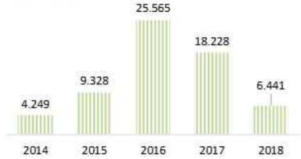
Yıllara Göre Yağmursuyu Kanal Uzunluğu (m)
